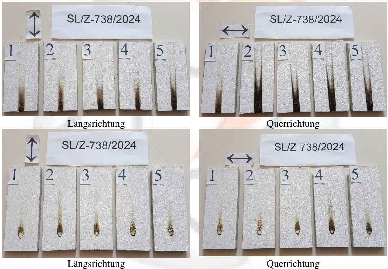
Bild 4. Aussehen des Probekörpers nach der Untersuchung
